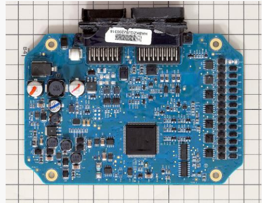
電池ECU基板外観
