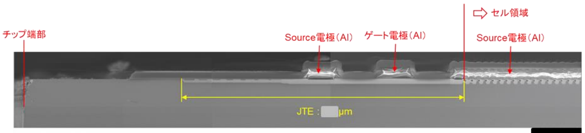
チップ外周部 断面SEM像
