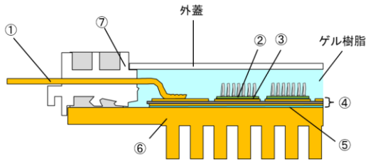
モジュール構造模式図
