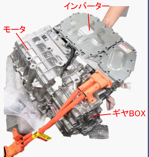
搭載e-Axle外観図(左:外観、右:カバー外し後)
