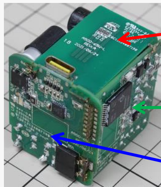
製品内観
