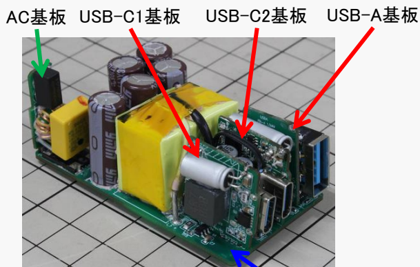
製品内観
