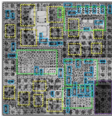
高周波モジュールX線画像
