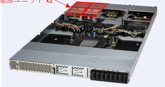
Nvidia GH200サーバユニット
