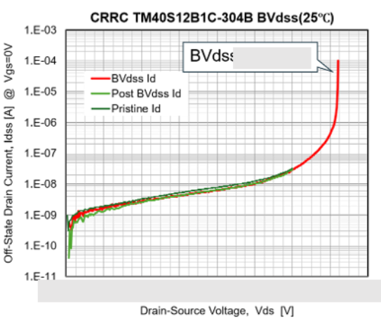
Fig.2-3-1 オフ状態破壊電圧BVdss
