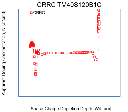
Fig. 2-9-1(a)深さ方向のキャリア濃度プロファイル
