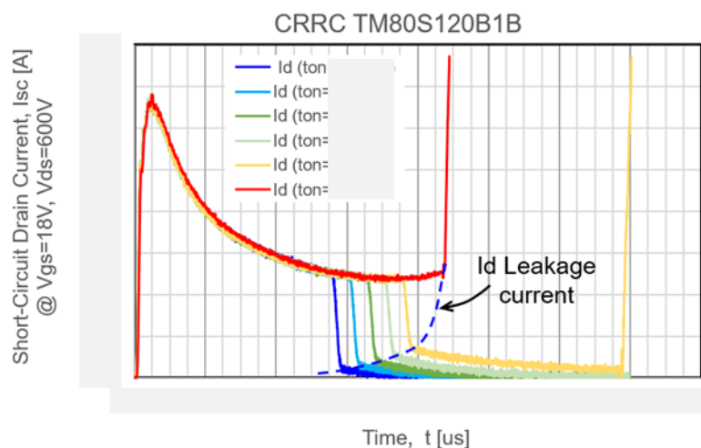
Fig.4-4-1 ゲート電圧ターンオン時間 ( t_{on}=2.0\mu s\sim 20\mu s ) に対する短絡ドレイン電流波形
