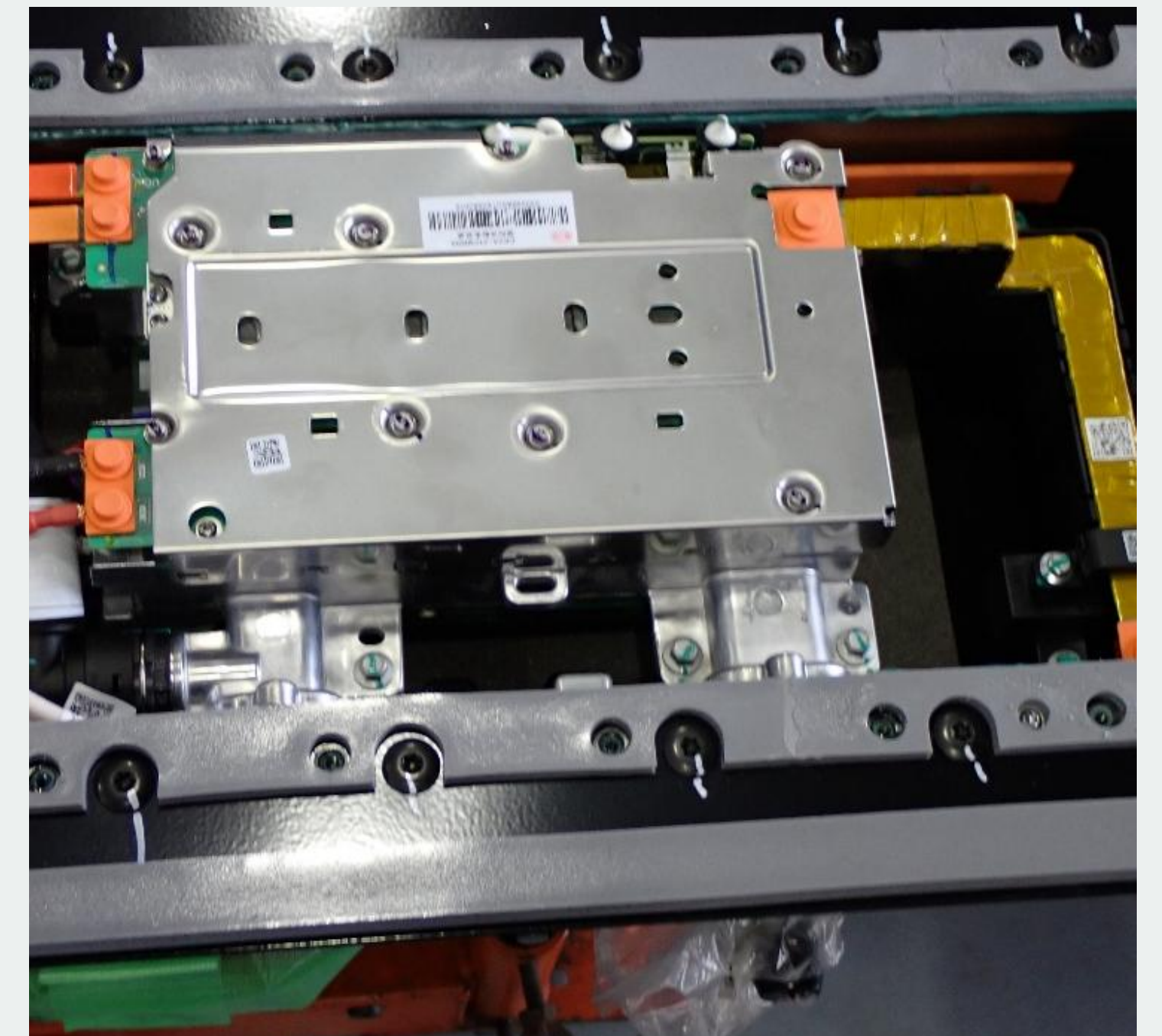
OBC+DCDC ※分解対象
