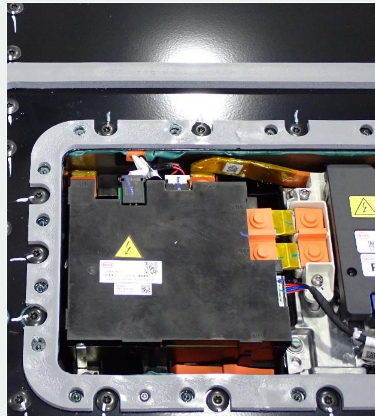
Junction BOX（PTC制御含む） ※分解対象
