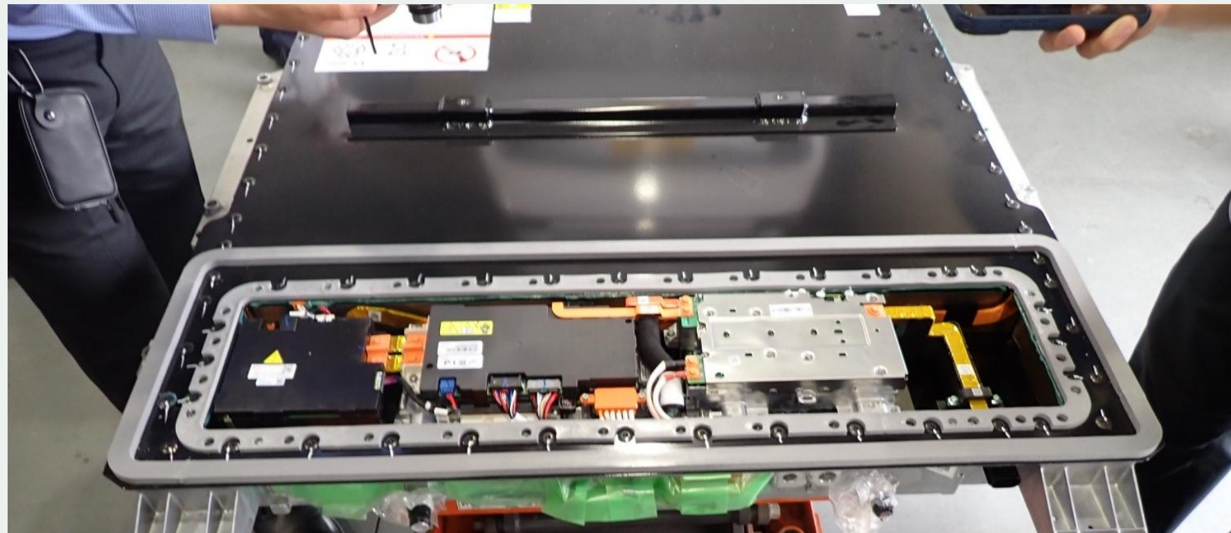
搭載電池パック(X-Pack) ※分解対象
