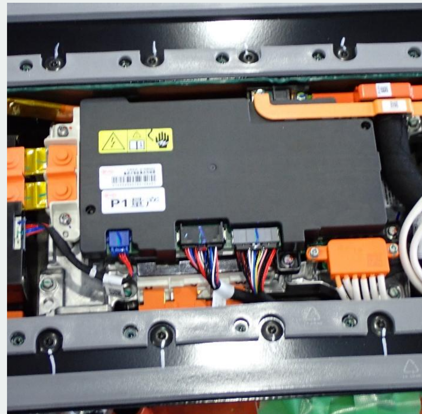
Inverter（MG & Comp） ※分解対象
