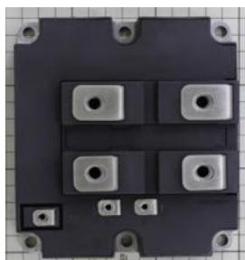
⑤ CM2400HC-34X モジュール外観
